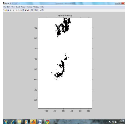
Fig.5. RFLICM output
